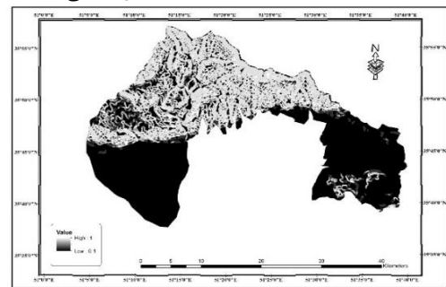
شکل ۷. فازی سازی طبقات شیب.
