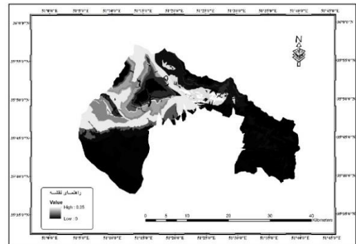
در نقشه‌ی AHP شکل ۱۳. تأثیر وزن مدل فازی سازی شده‌ی طبقات لیتولوژیکی.
