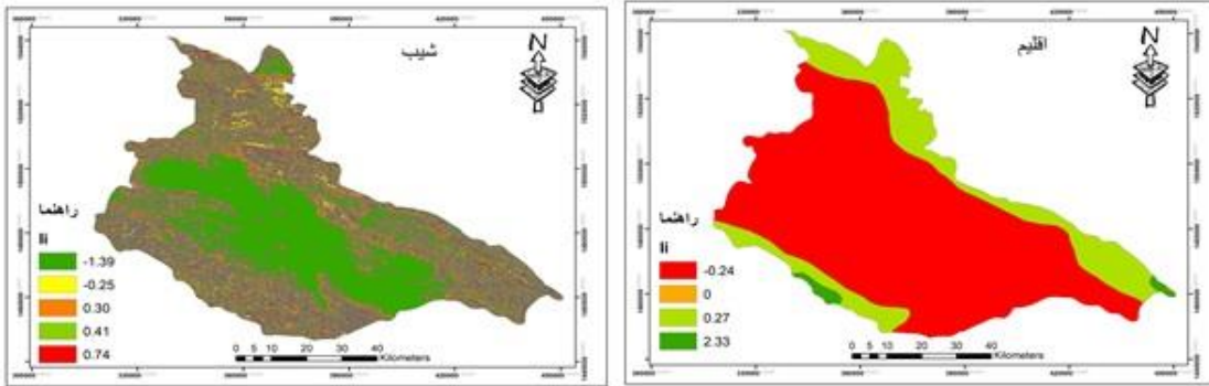
(۴) پهنه‌بندی لغزش بر اساس عامل شیب
