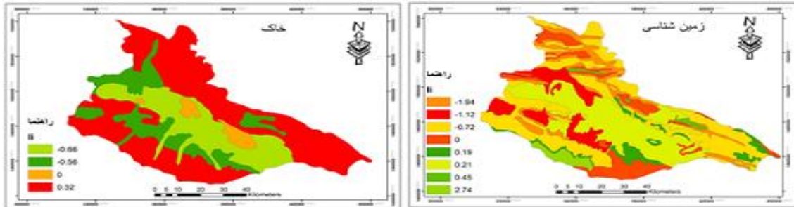
(۶) پهنه‌بندی لغزش بر اساس عامل خاکشناسی
