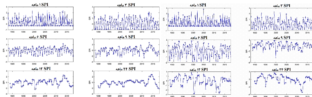
شکل ۱۲. SPI ایستگاه اعقدا
