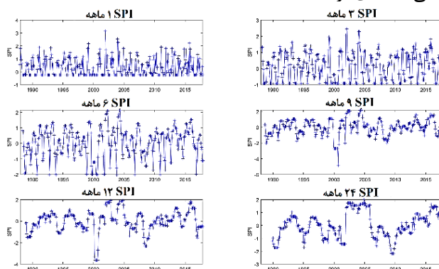
شکل ۱۳. SPI ایستگاه ابرکوه
