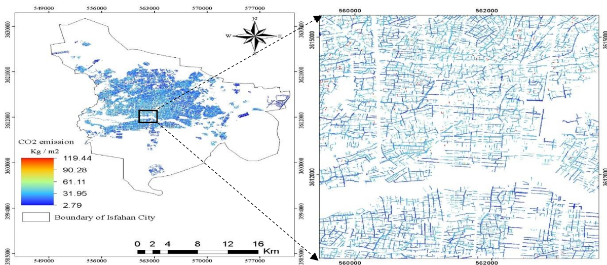
شکل ۵. نقشه توزیع مکانی انتشار سالیانه گاز CO 2 ناشی از احتراق سوخت‌های فسیلی از خودروهای سبک در خیابان-
