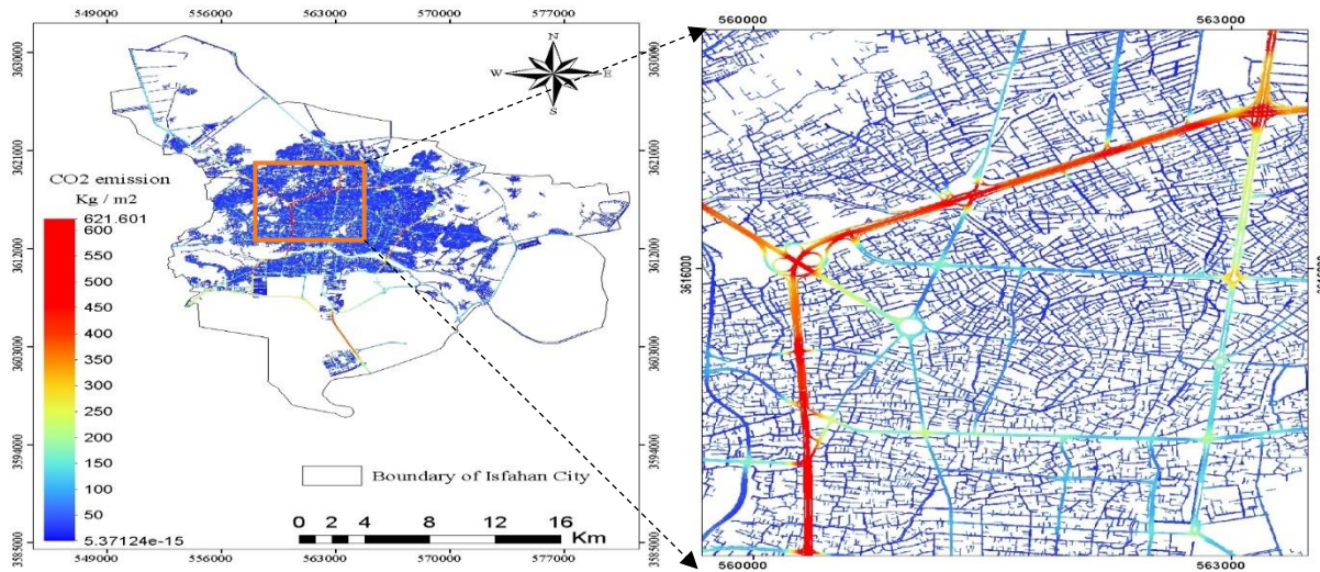
شکل ۴. نقشه توزیع مکانی انتشار سالیانه گاز CO 2 ناشی از احتراق سوخت‌های فسیلی از خودروهای سبک در خیابان-
