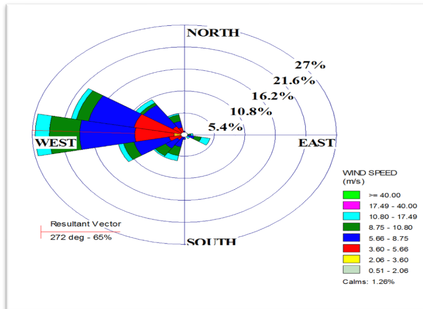
شکل ۵- گلغبار بلندمدت ایستگاه سینوپتیک لردگان ۱۹۹۵-۲۰۱۹
