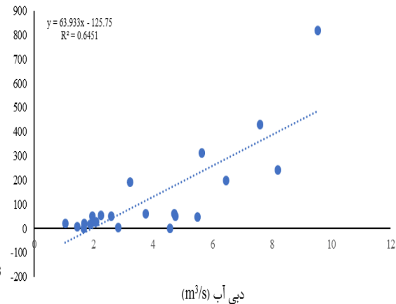
شکل ۱۰. منحنی سنج رسوب ایستگاه گلورد (فصل بهار)
