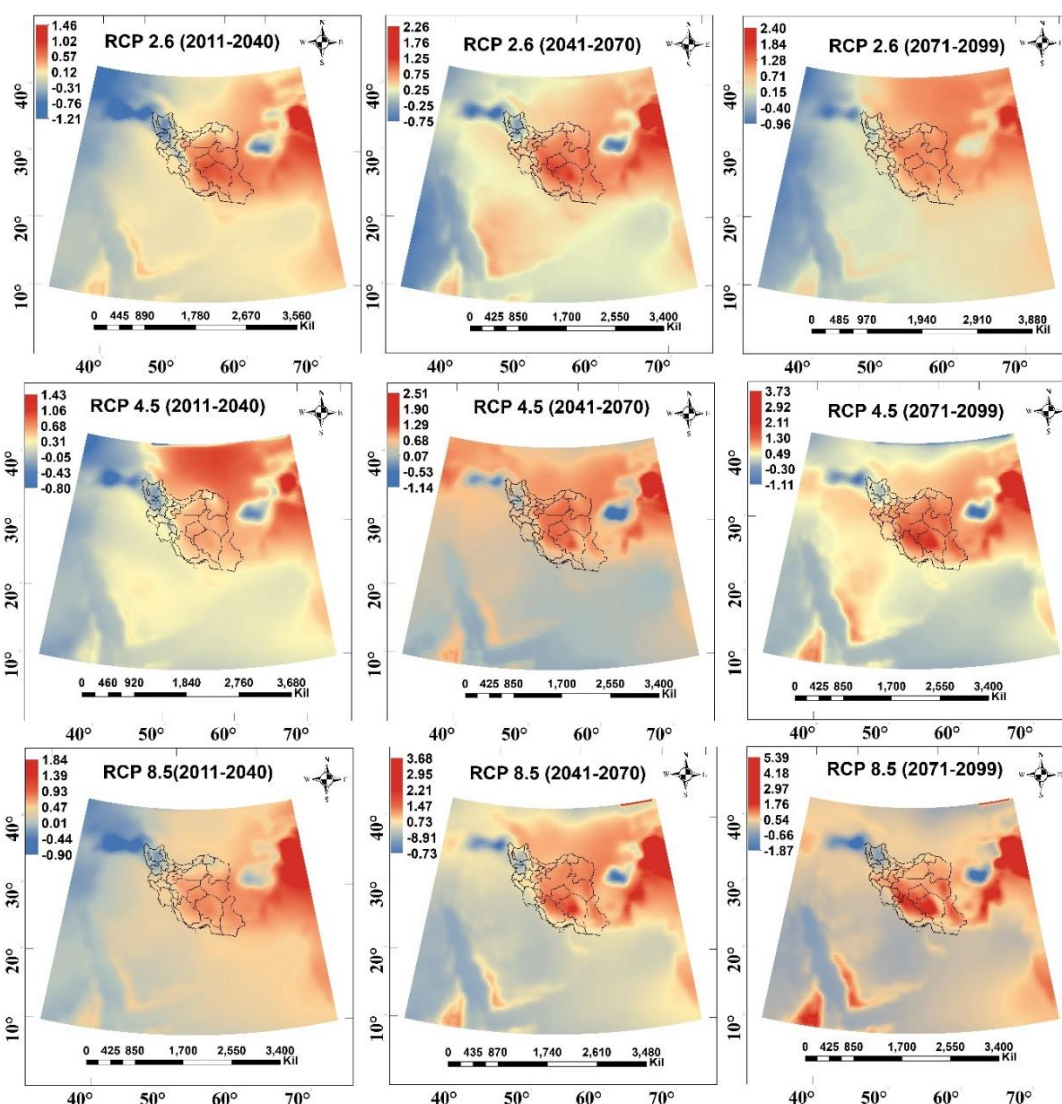
شکل ۵- ناهنجاری فشار (بر واحد هکتوپاسکال) تراز دریا (SLP) فصل زمستان طی دوره آینده نزدیک (۲۰۱۱-۲۰۴۰)، آینده میانی (۲۰۴۱-۲۰۷۰) و آینده دور (۲۰۷۱-۲۰۹۹) بر اساس مدل HadGEM ۲ -ES تحت سناریوهای واداشت تابشی (RCPs)
