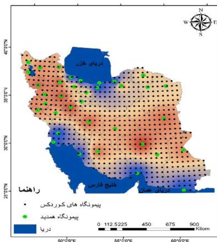
شکل ۱. موقعیت منطقه مورد مطالعه به همراه پیمونگه های همید منتخب و یاخته های CORDEX- WAS با قدرت تفکیک مکانی ۰/۴۴ درجه قوسی
