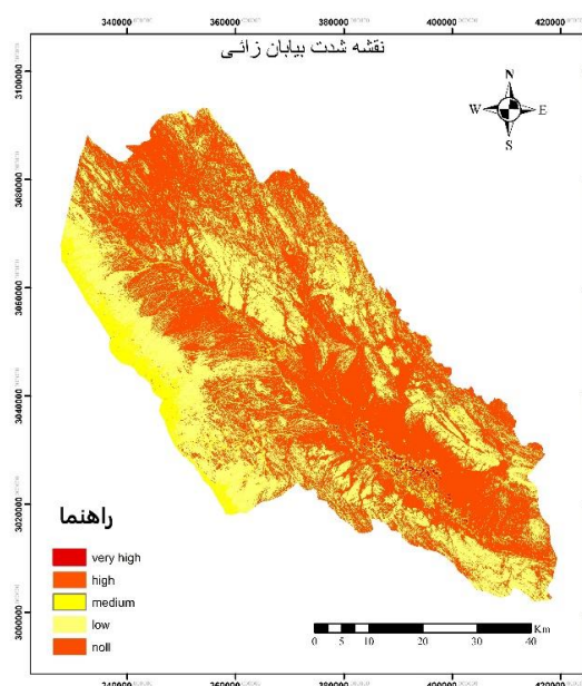
شکل (۵). نقشه شدت بیابان‌زایی حاصل از معادله I = a * \text{NDVI} - \text{Albedo}
