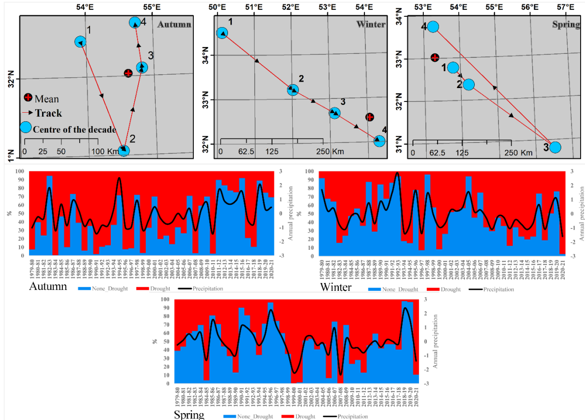
شکل ۸. موقعیت مکانی میانگین دهه‌ی مرکز ثقل خشکسالی ایران براساس شاخص RAI (شمارش معرف هر دهه است)، همراه با سری زمانی تغییرات درصد مساحت گستره خشکسالی در طی بازه ۴۲ ساله (۱۹۷۹-۲۰۲۱)، محور راست آنومالی بارش و محور چپ درصد گستره خشکسالی
