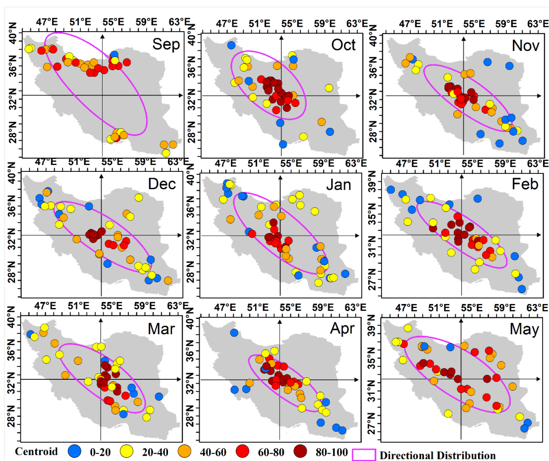
شکل ۵. مراکز ثقل (دوایر رنگی بر حسب درصد گستره خشکسالی) و توزیع جهت‌دار خشکسالی‌های ماهانه ایران (۱۹۷۹-۲۰۲۱)
