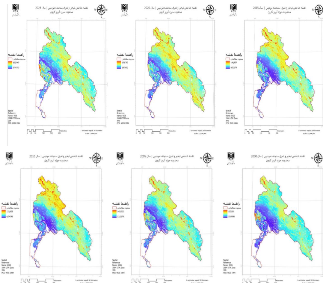
شکل ۱۷. نقشه های شاخص تبخیر و تعرق حوزه آبریز کارون، میانگین سالانه ۲۰۰۰ تا ۲۰۲۳
